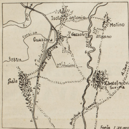
Schizzo planimetrico dei due tracciati allo studio.
